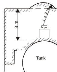
Bereich der Ladung oberhalb des Decks für verschiedene Tankschiffe
