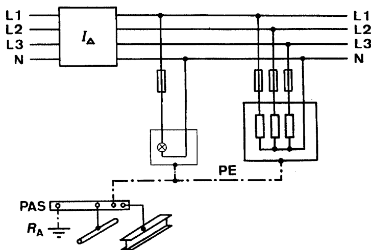
Bild 12-1: Fehlerstrom-Schutzschaltung als Fehlerschutz gemäß 3.8.13
