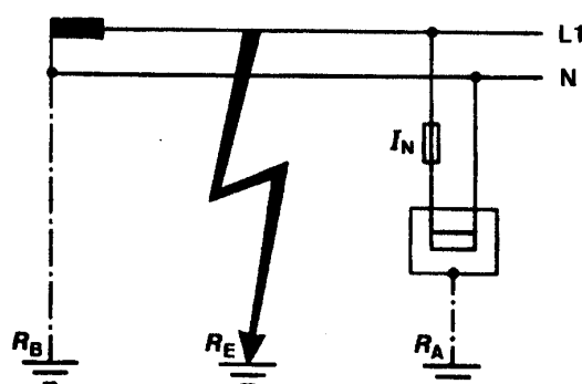
Bild 14-1: Erdschluss in einem geerdeten Verteilungsnetz und einer Verbraucheranlage im TT-System
