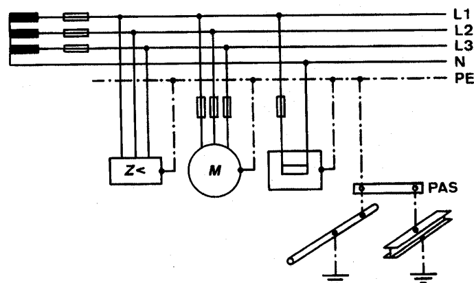
Bild 11-1: Beispiel für ein Isolationsüberwachungssystem
