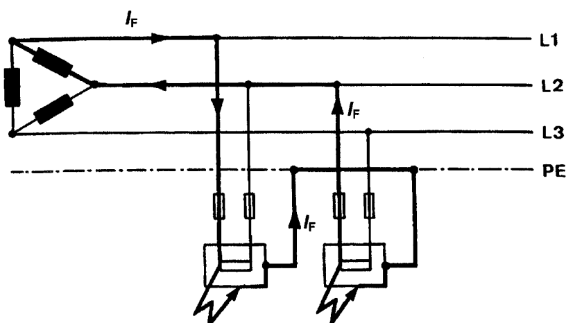
Bild 11-2: Fehlerstromkreis bei Körperschluss an zwei Geräten
