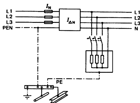
Bild 10-2: Fehlerstrom-Schutzeinrichtung zur Erfüllung der Ausschaltbedingung gemäß 10.2.1.3
