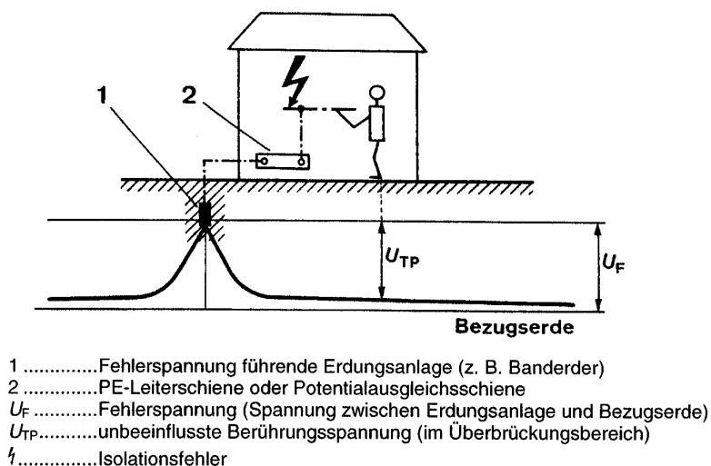
Bild 3-8: Zusammenhang zwischen Fehlerspannung U_F und unbeeinflusster Berührungsspannung U_{TP}
