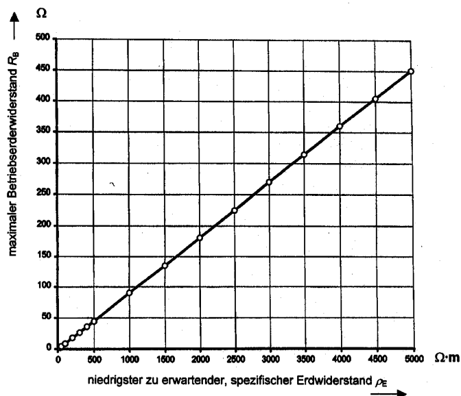
Bild 14-2-1: Maximal zulässiger Wert für den Gesamterdwiderstand aller Betriebserder R_B in Abhängigkeit vom niedrigsten zu erwartenden, spezifischen Erdwiderstand \rho_E für U_N = 230 V
