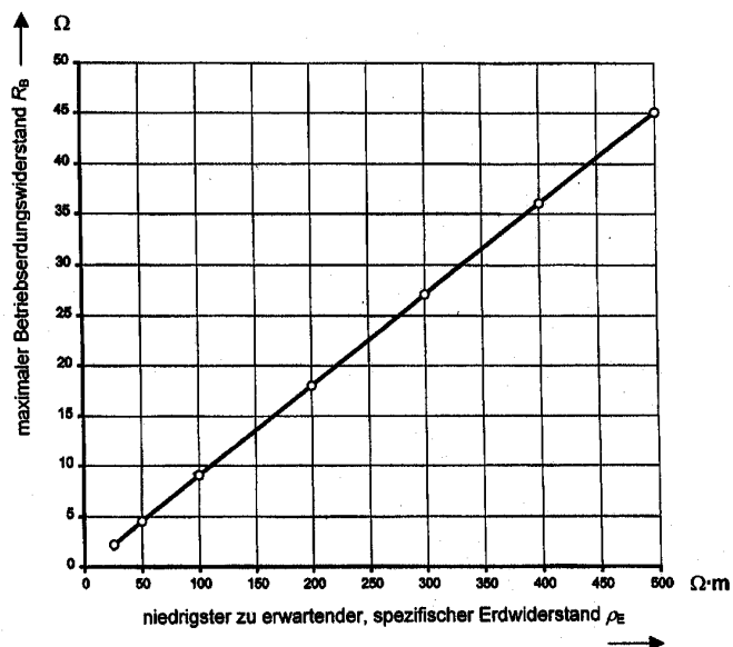
Bild 14-2-2: Maximal zulässiger Wert für den Gesamterdwiderstand aller Betriebserder R_B in Abhängigkeit vom niedrigsten zu erwartenden, spezifischen Erdwiderstand \rho_E (Detailbereich bis 500 \Omega \cdot m ) für U_N = 230 V
