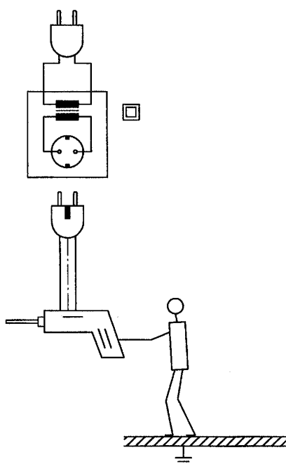
Bild 13-1: Schutztrennung mit einem angeschlossenen Betriebsmittel
