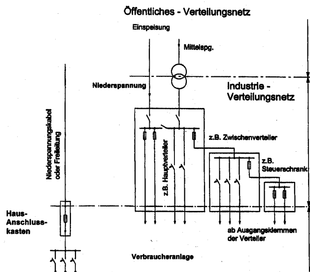
Bild 3-6: Beispiele für die Abgrenzung Verbraucheranlage und Verteilungsnetz
