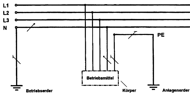
Bild 3-4: TT-System
