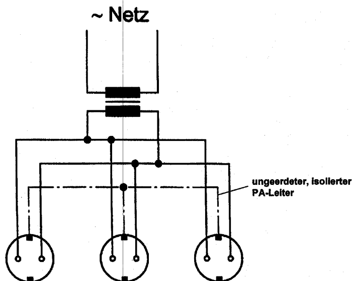
Bild 13-2: Schutztrennung mit mehreren angeschlossenen Betriebsmitteln
