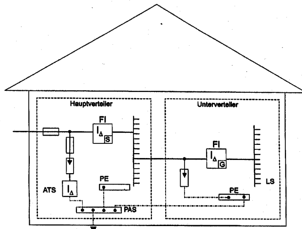
Bild 18-7: Beispiel für die zulässige Anordnung von Überspannungs-Schutzeinrichtungen der Ableiterklasse C bzw. der Prüfklasse II nach einer Fehlerstrom-Schutzeinrichtung
