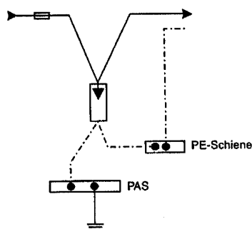
Bild 18-10: V-förmiger Anschluss der Zuleitung (und Erdungsleitung)
