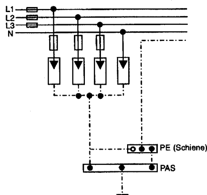
Bild 18-8: Anordnung der Überspannungs-Schutzeinrichtungen in IT-Systemen gemäß (1) a)
