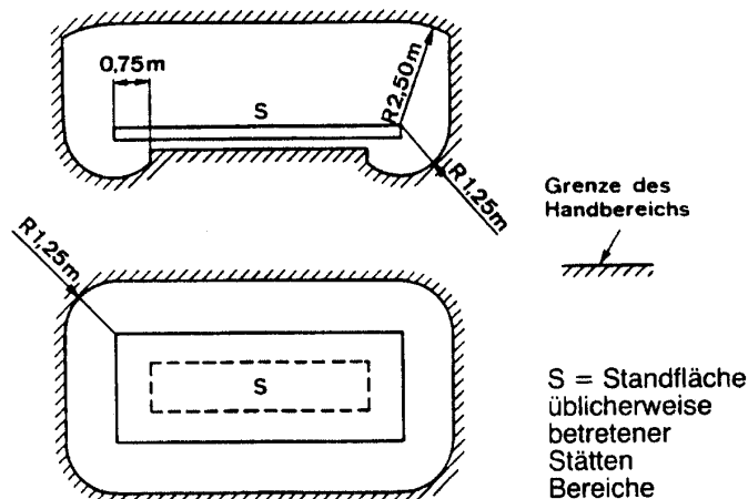
Bild 3-14: Maße des Handbereiches
