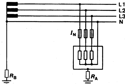
Bild 9-1: Schutzterdung
