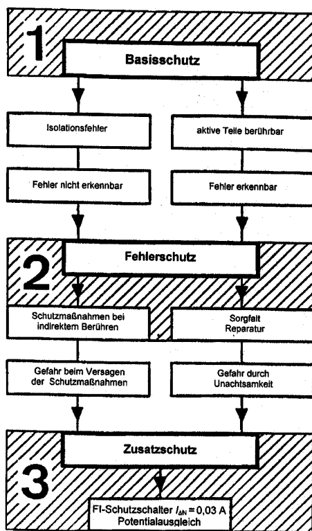
Bild 3-13: Maßnahmen für den Schutz gegen elektrischen Schlag
