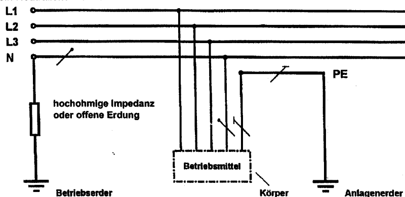
Bild 3-5: IT-System
