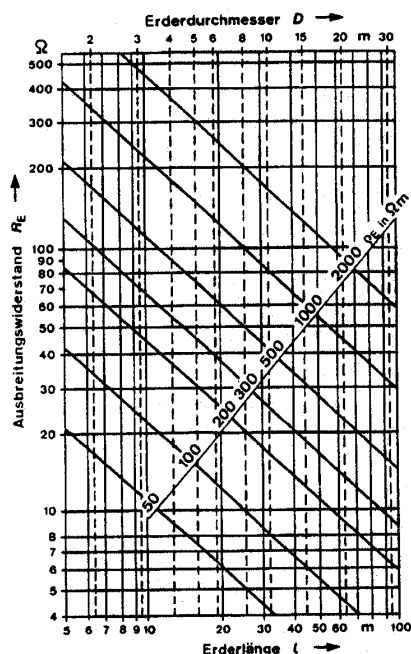
Bild 20-1: Ausbreitungswiderstand R_E von Horizontalerden (aus Band, Rundmaterial oder Seil) bei gestreckter Verlegung in Abhängigkeit von der Länge l und von Maschenerden entsprechend einem Durchmesser D bei verschiedenen spezifischen Erdwiderständen \rho_E
