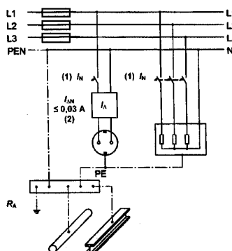
Bild 6-1: Nullung mit Zusatzschutz durch eine Fehlerstrom-Schutzeinrichtung mit einem Nennfehlerstrom I_{\Delta N} \leq 0,03 \text{ A}
