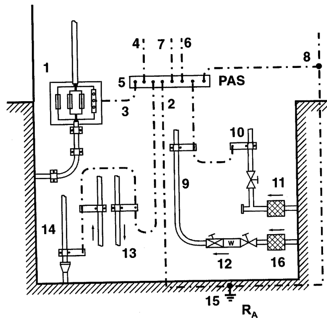
Bild 15-1: Beispiel für Hauptpotentialausgleich mit Haupterdungsschiene (PAS) und Potentialausgleichsleitern
