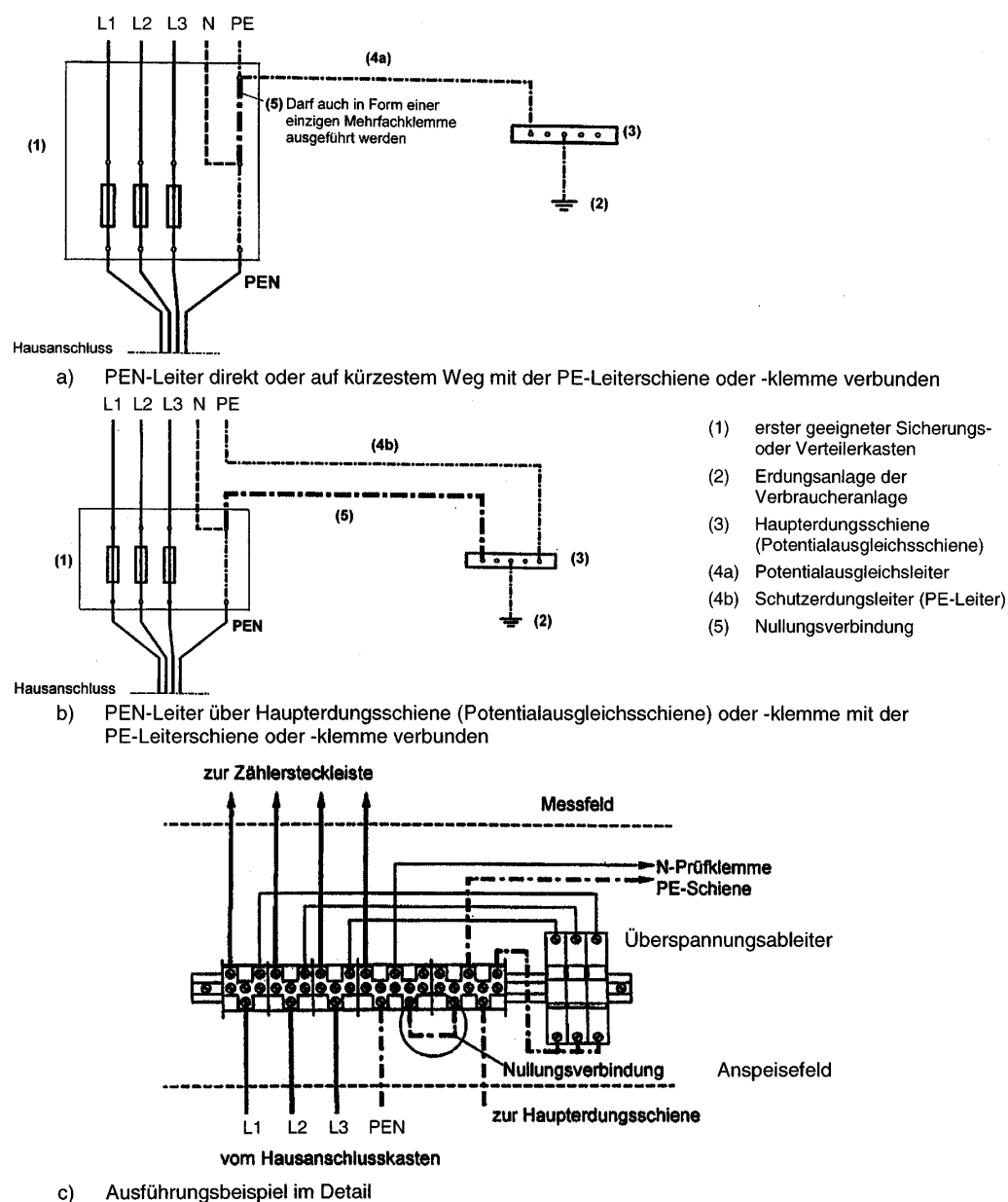
Bild 10-1: Beispiele für die Anordnung der Nullungsverbindung
