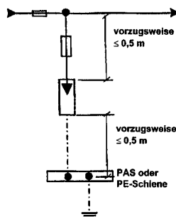
Bild 18-9: Impedanzarme, kurze ÜSE-Zuleitungen und Erdungsleitungen
