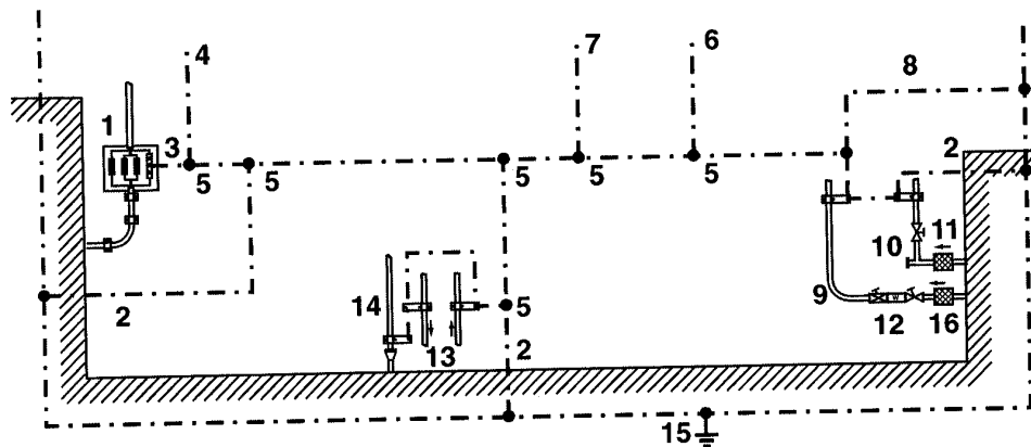
Bild 15-1: Beispiel für Hauptpotentialausgleich mit Haupterdungsschiene (PAS) und Potentialausgleichsleitern
