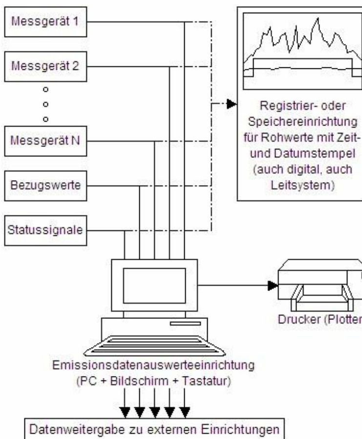
Bild 1 — Methoden zur Auswertung kontinuierlicher Emissionsmessungen
